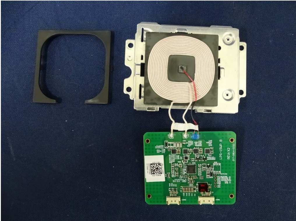
(15) EUT Photo
