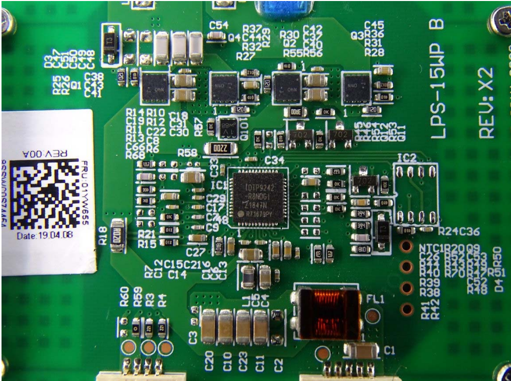
(21) EUT Photo
