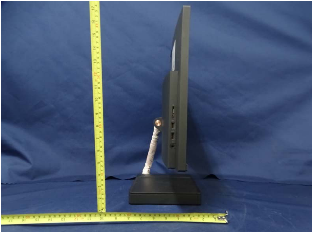
(42) EUT Photo _ IdeaCentre AIO 5 24IMB05
