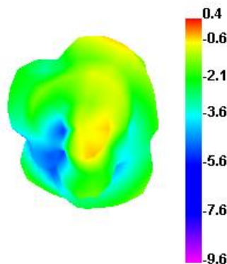
2500.000MHz E1
