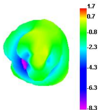
2450.000MHz E1
