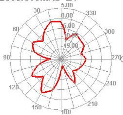
2500.000MHz E1
