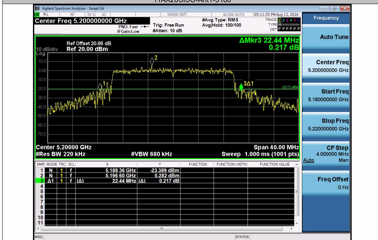
11AX20SISO-Ant1-5200
