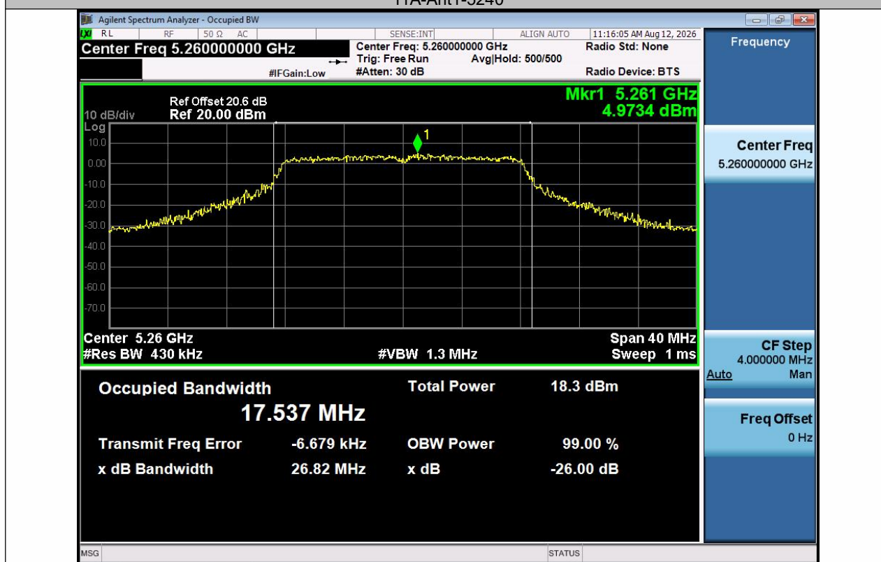
11A-Ant1-5260
