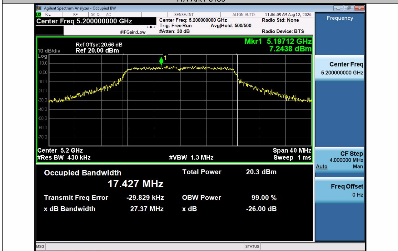
11A-Ant1-5200
