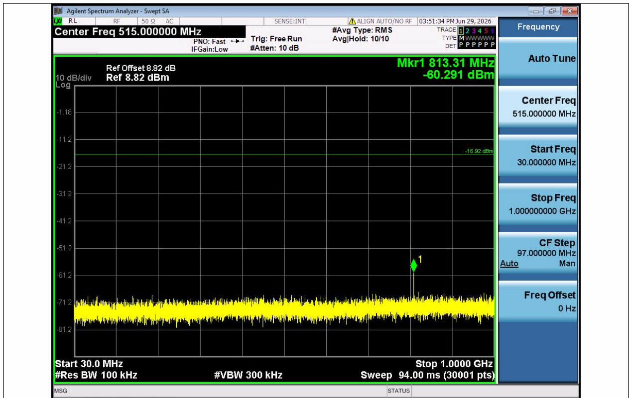
BLE 1M-Ant1-2440-30~1000-PASS
