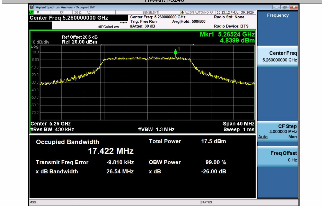
11A-Ant1-5260
