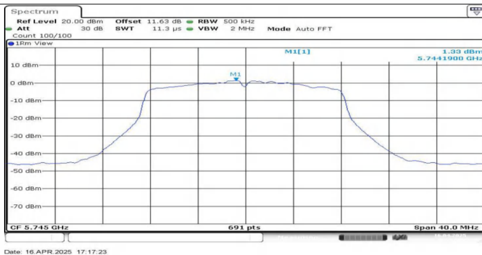
11A-Ant1-5745
