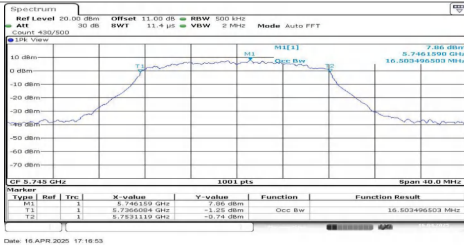
11A-Ant1-5745
