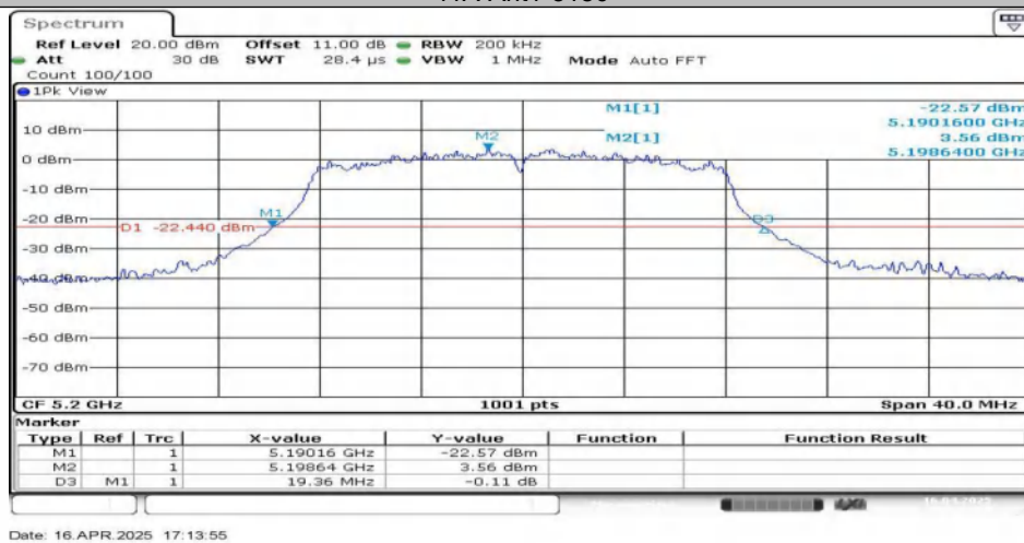
11A-Ant1-5200
