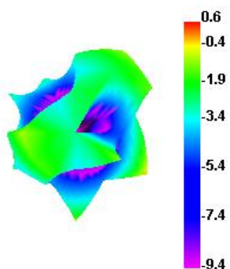
5150.000MHz E1
