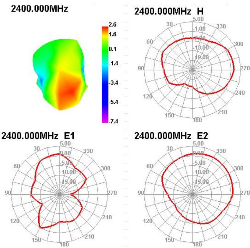
3D 方向图
