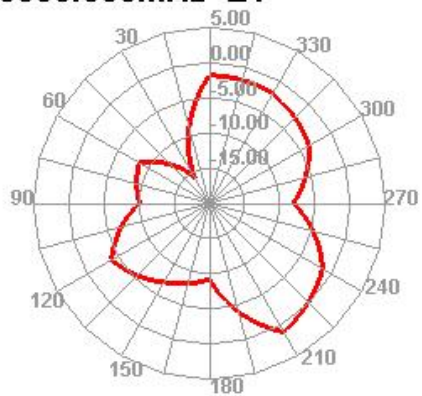
5550.000MHz E1
