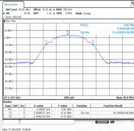
11B-Ant1-2437
