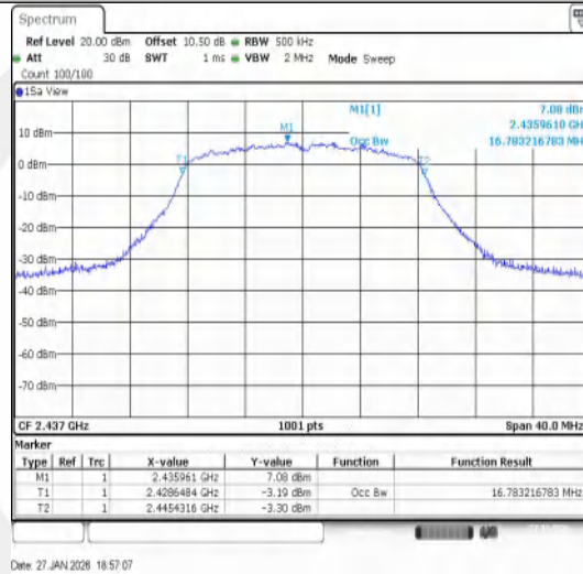
11G-Ant1-2437
