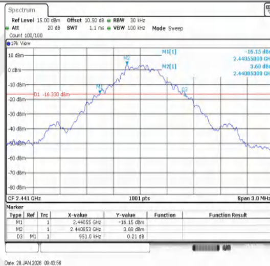
DH5-Ant1-2441
