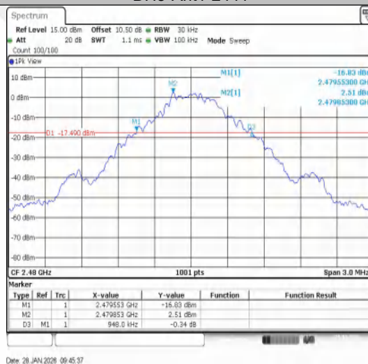
DH5-Ant1-2480
