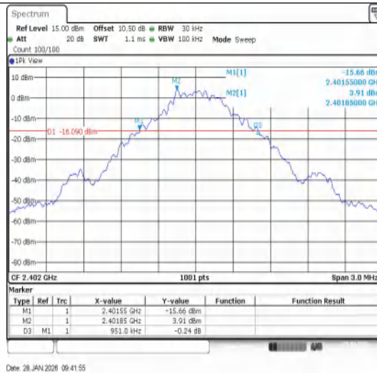
DH5-Ant1-2402
