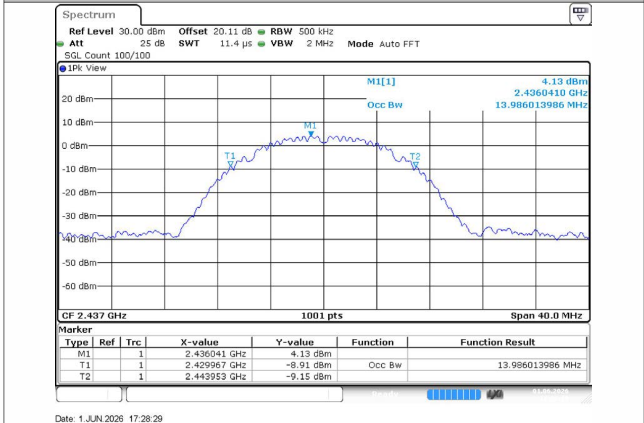
11B-Ant1-2437
