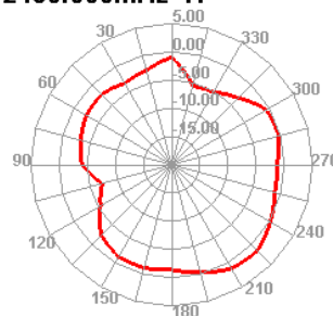
2480.000MHz H
