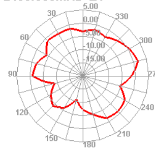
2480.000MHz E1
