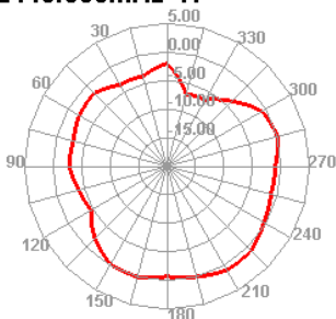
2440.000MHz H
