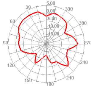
2440.000MHz E2
