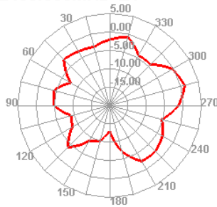
2440.000MHz E1
