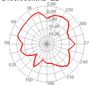
2480.000MHz E2
