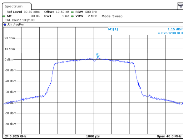
802.11ac20_5825MHz_Chain 0
