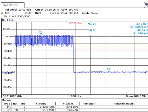
DH1_Hopping_Upper
