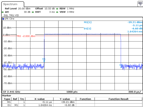
DH3_Hopping 1.643ms
