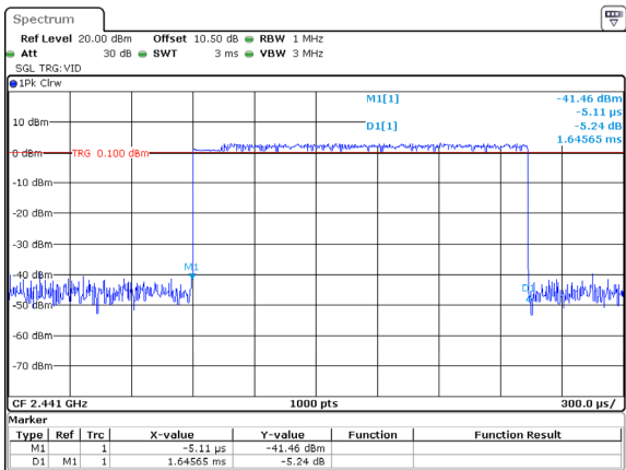
2DH3_Hopping 1.646ms
