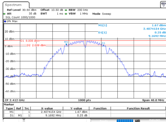
802.11b_2412MHz_Chain 0
