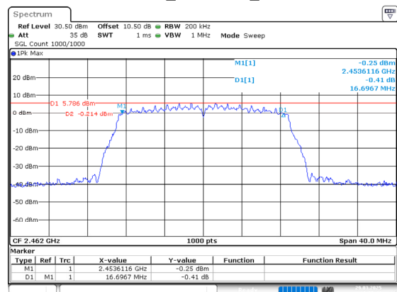
802.11n20_2462MHz_Chain 1
