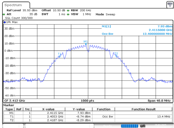
802.11b_2412MHz_Chain 0
