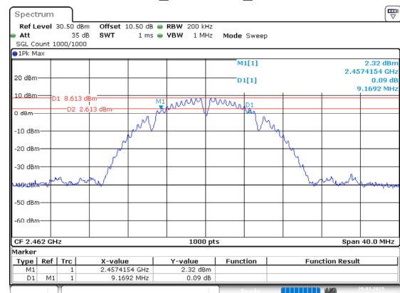
802.11b_2462MHz_Chain 1
