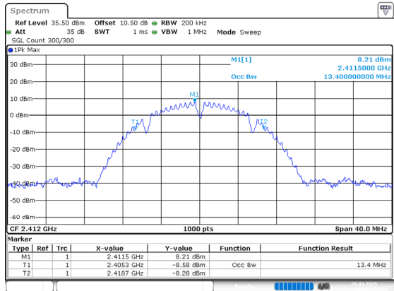
802.11b_2412MHz_Chain 1
