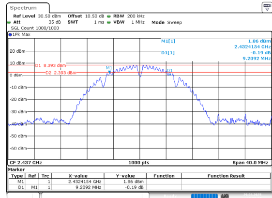
802.11b_2437MHz_Chain 0
