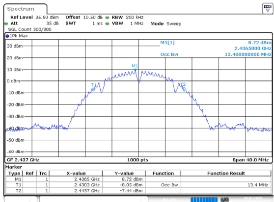
802.11b_2437MHz_Chain 1
