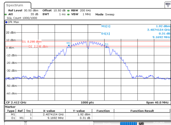
802.11b_2412MHz_Chain 1
