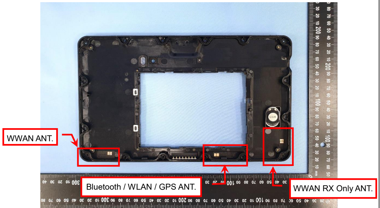
EUT Photo (2)
