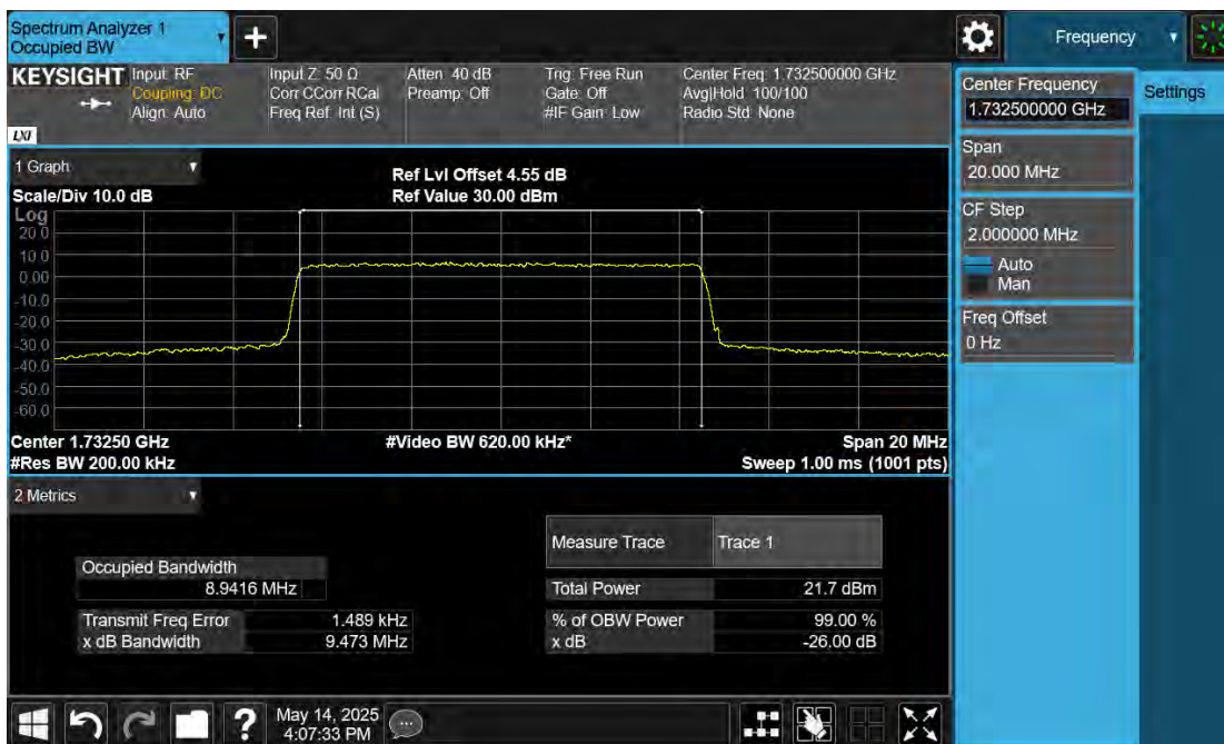
B4\Band4-10MHz-QPSK-20175-50RB#0
