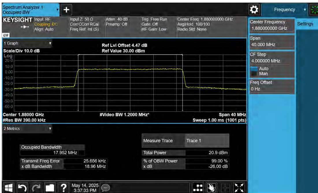
B2\Band2-20MHz-16QAM-18900-100RB#0
