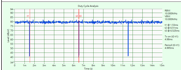
802.11n (HT20)
