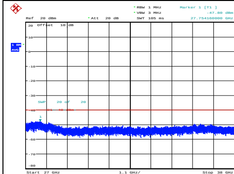
B48-20-10-CSE-L-Q64-3
