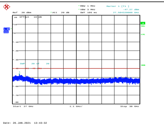
B48-10-20-CSE-H-QPSK-2
