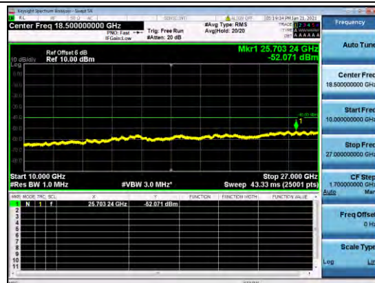
B48-10M-CSE-L-Q64-1
