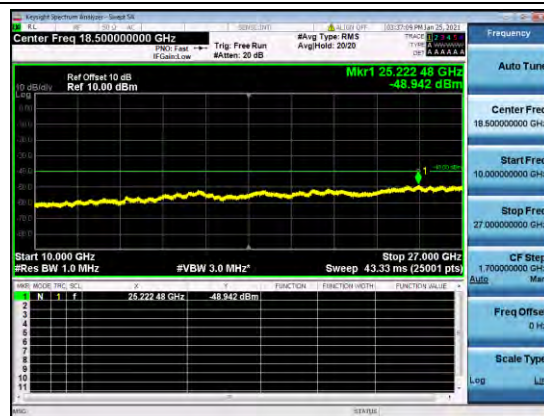
B48-20-10-CSE-M-QPSK-1
