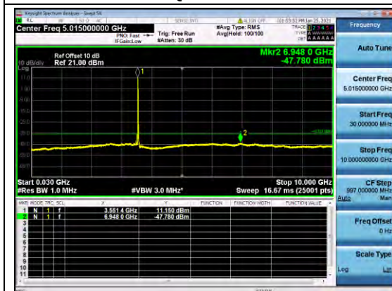
B48-15-20-CSE-L-Q16-3
