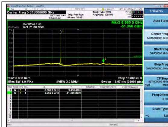
B48-15M-CSE-H-QPSK-3
