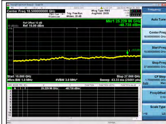
B48-20-10-CSE-L-Q64-1
