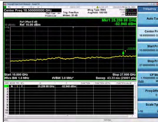
B48-5M-CSE-H-Q16-1
