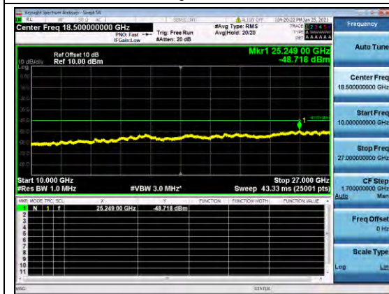
B48-20-10-CSE-H-Q64-1
