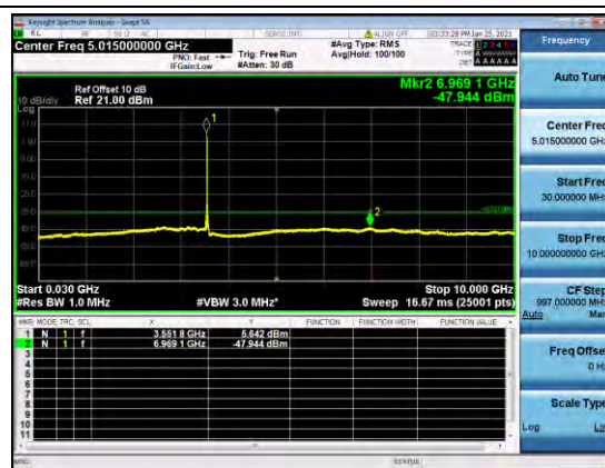
B48-20-10-CSE-L-Q16-3
