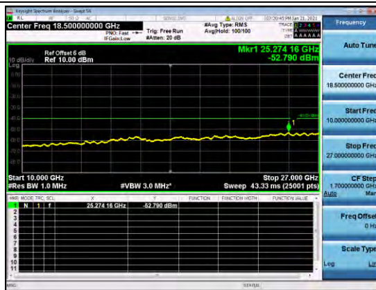
B48-20M-CSE-L-QPSK-1
