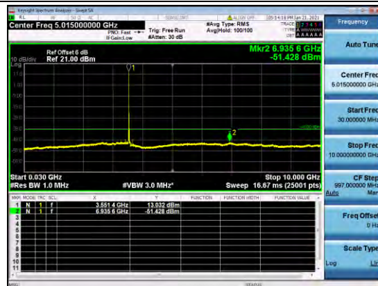
B48-10M-CSE-L-QPSK-3
