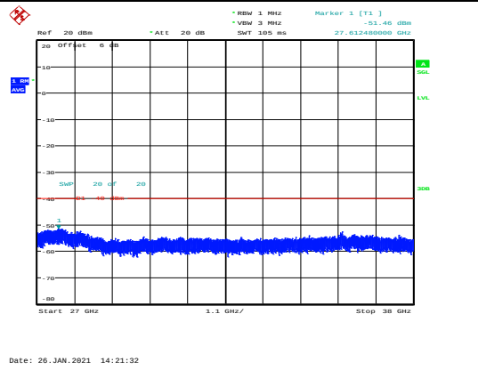
B48-5M-CSE-H-Q64-2
