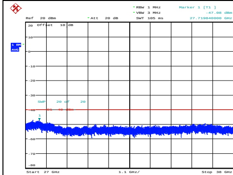
B48-15-20-CSE-M-QPSK-3
