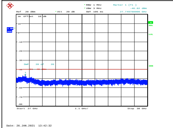
B48-15-20-CSE-L-QPSK-2
