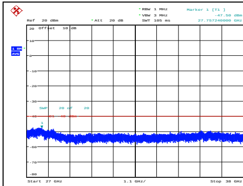
B48-15-20-CSE-L-Q64-2
