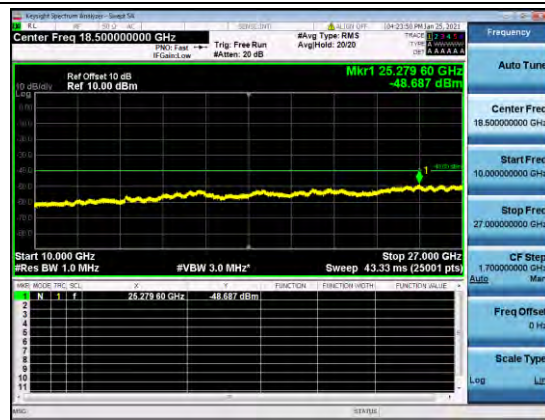
B48-20-15-CSE-L-QPSK-1
