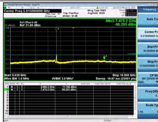
B48-5M-CSE-H-Q16-3
