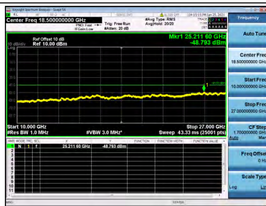
B48-20-10-CSE-H-Q16-1
