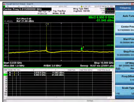
B48-15M-CSE-M-Q64-1
