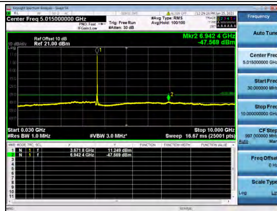
B48-10-20-CSE-H-Q16-3
