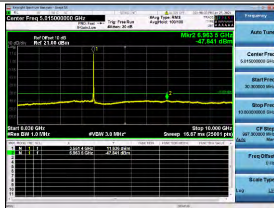
B48-15-20-CSE-L-QPSK-3
