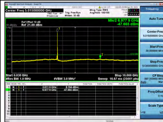
B48-15-20-CSE-M-Q16-3
