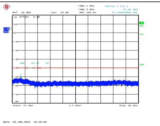
B48-5M-CSE-H-QPSK-2
