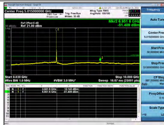
B48-20M-CSE-L-Q64-2
