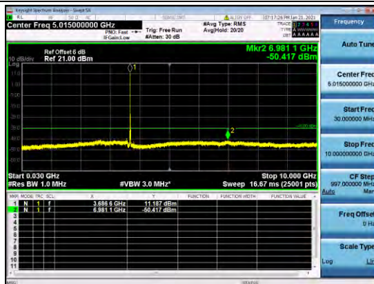
B48-15M-CSE-H-Q16-3
