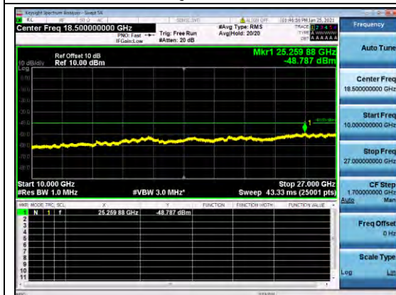
B48-15-20-CSE-L-Q16-1
