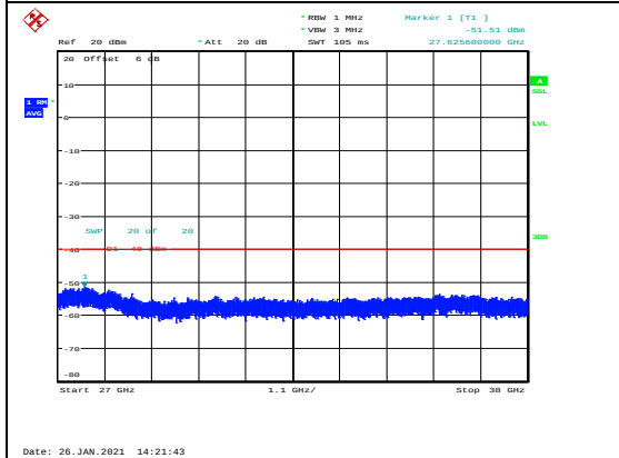
B48-10M-CSE-L-QPSK-2
