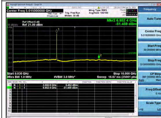
B48-10M-CSE-L-Q16-3
