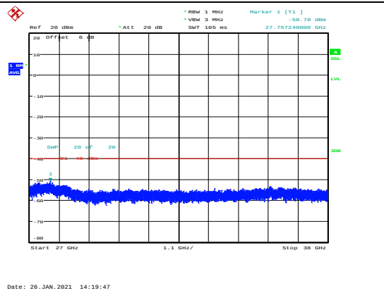
B48-15M-CSE-H-QPSK-2
