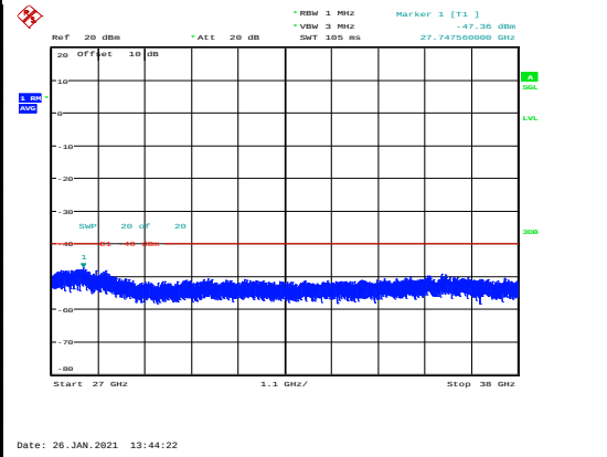
B48-15-20-CSE-M-QPSK-2
