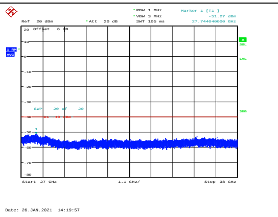
B48-15M-CSE-M-Q16-2
