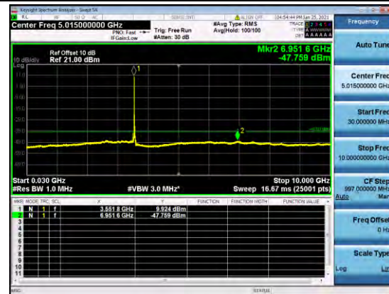
B48-20-15-CSE-L-Q64-3
