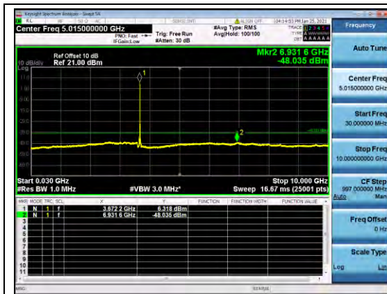
B48-20-10-CSE-H-QPSK-3
