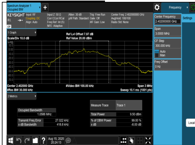
IC OBW_BLE 1M_LowCH00-2402MHz
