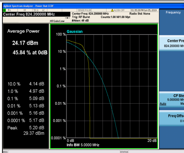
EGPRS850_128
