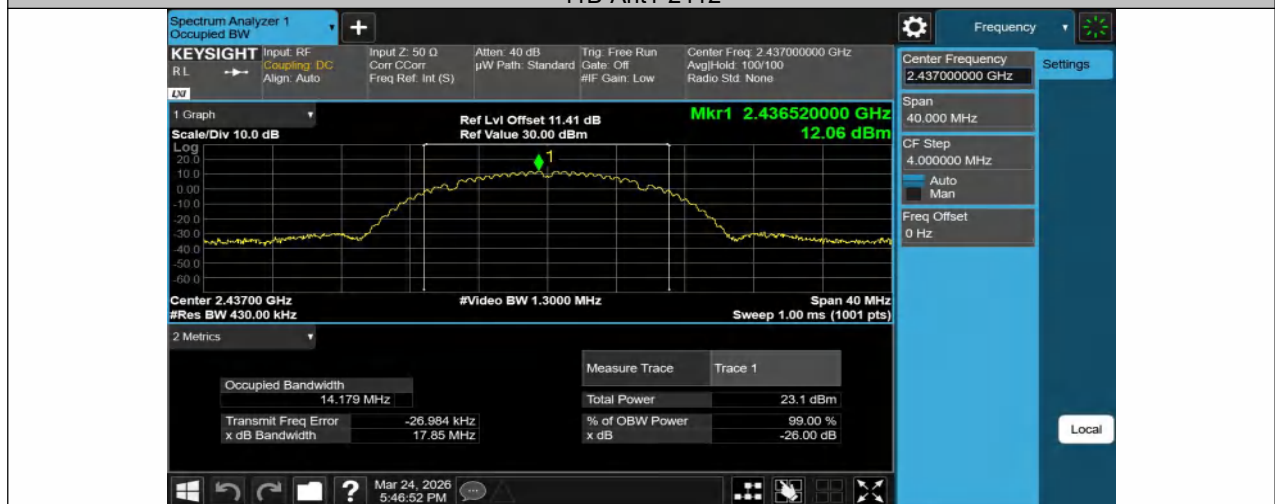
11B-Ant1-2437
