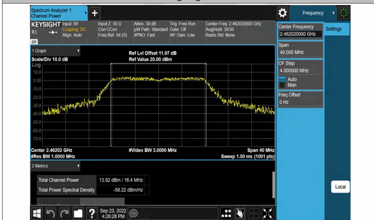
11G_Ant1_2462
