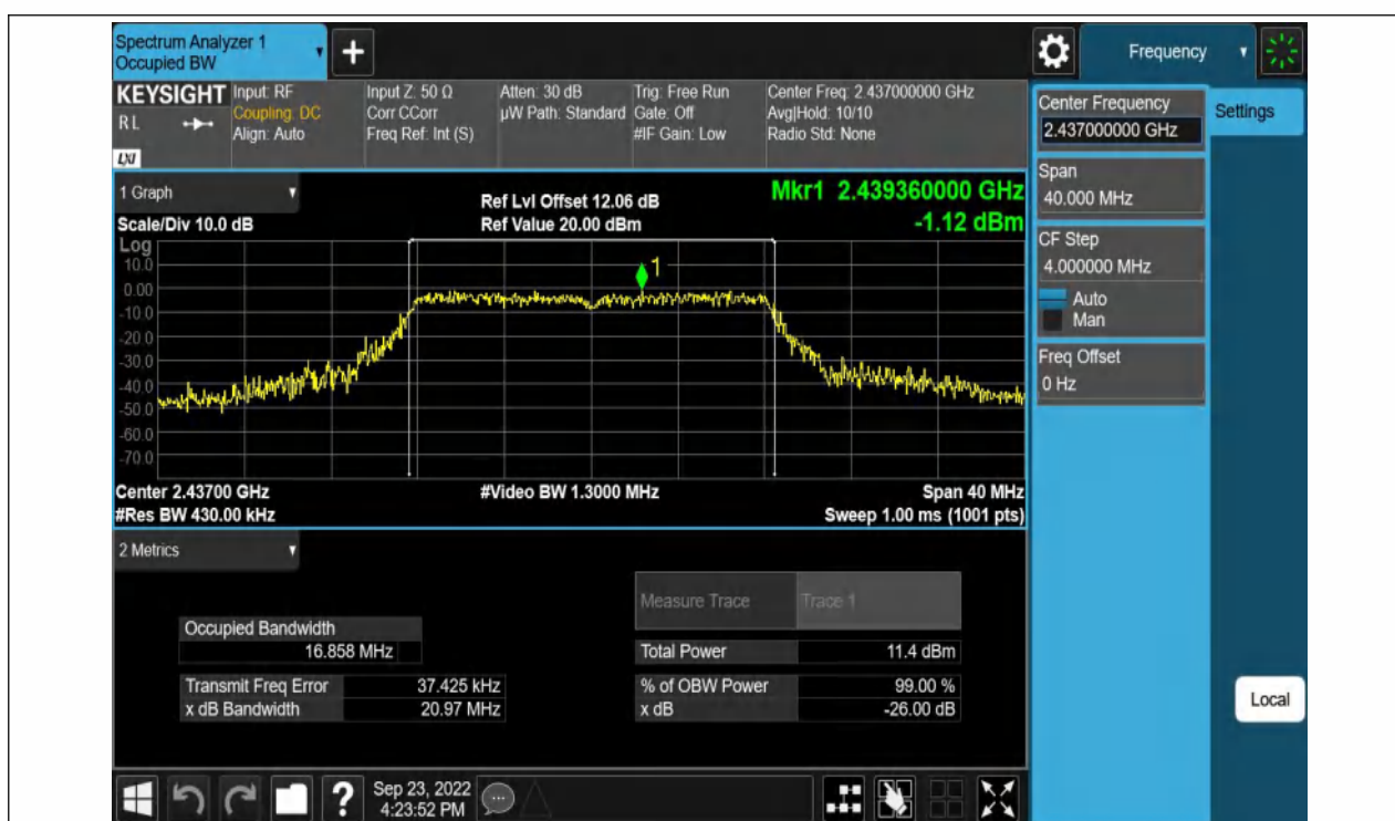
11G_Ant1_2437
