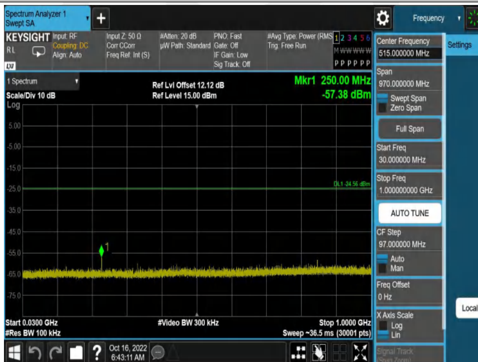
11B-Ant1-2412-30~1000
