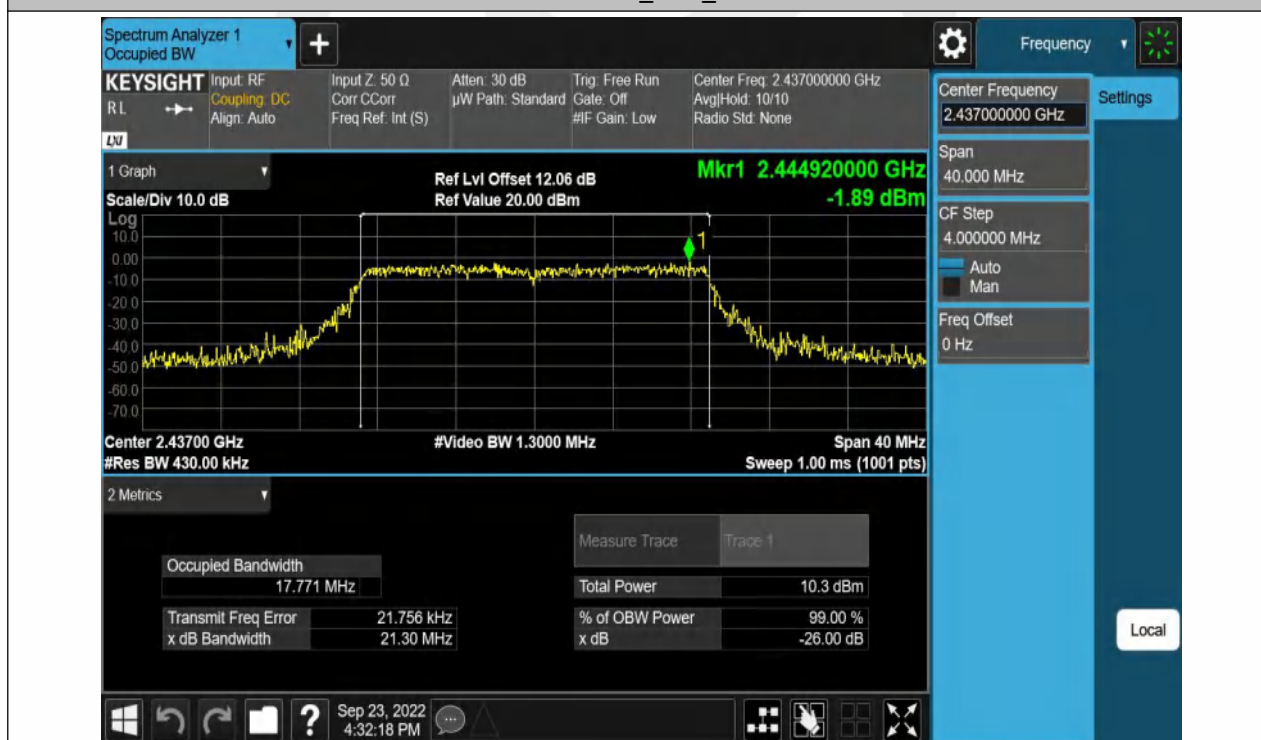
11N20SISO_Ant1_2437
