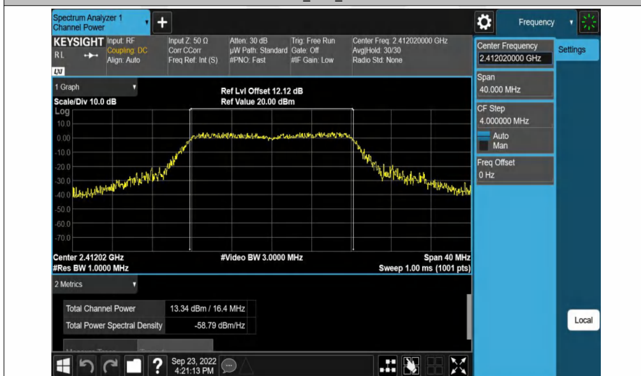
11G_Ant1_2412
