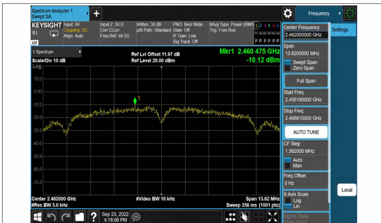
11B_Ant1_2462
