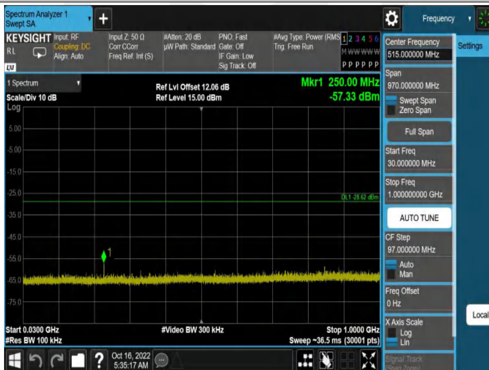
11G-Ant1-2437-30~1000
