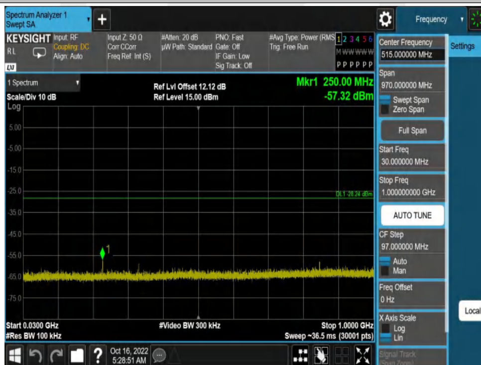
11G-Ant1-2412-30~1000
