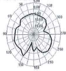
2500.000MHz E1
