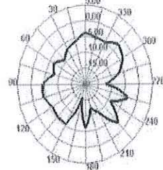
2475.000MHz E2
