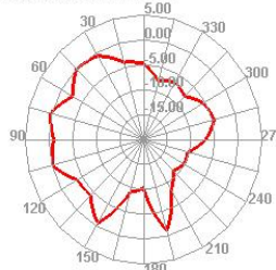
2500.000MHz E1
