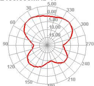
2400.000MHz H
