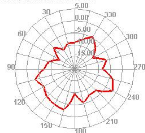
2450.000MHz E2
