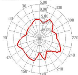
2500.000MHz E2
