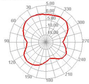
2450.000MHz H
