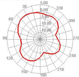
2500.000MHz H
