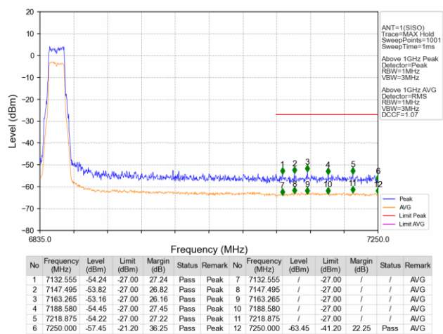
802.11ax(HEW20) HCH 6855MHz_SU / Ant1_NTNV
