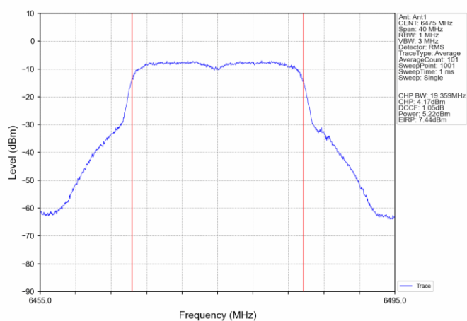
802.11ax(HEW20) MCH 6475MHz SU / Ant1_NTNV
