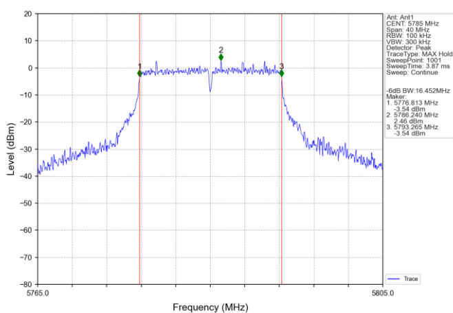
802.11a_MCH_5785MHz_Ant1_NTNV
