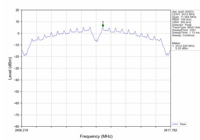
802.11b_LCH_2412MHz_Ant2 (SISO)_NTNV
