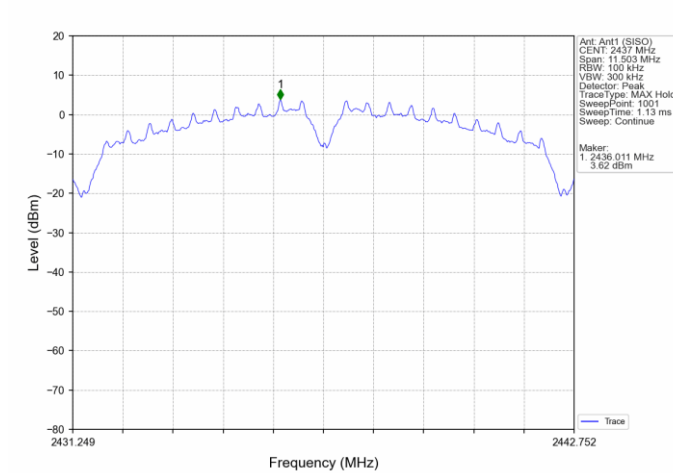
802.11b_MCH_2437MHz_Ant1 (SISO)_NTNV
