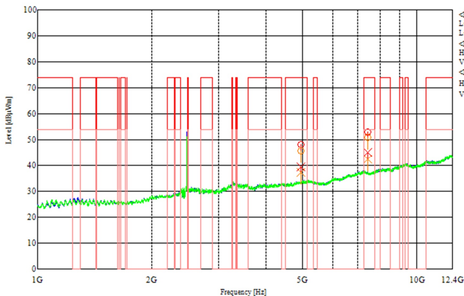
[Chart] Tx 2480MHz 2Mbps X-plane
