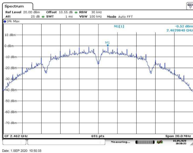
PSD, 2462 MHz, 802.11b, 1Mb
