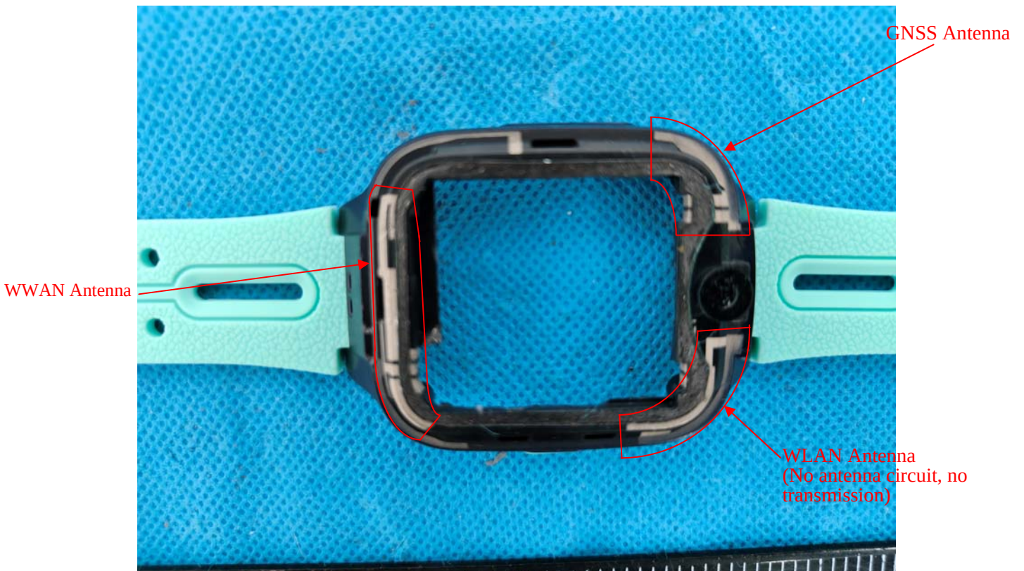
Antnena
