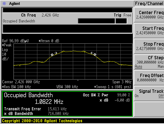
BLE mode 2426 MHz 6 dB OBW
