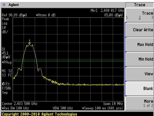
BLE mode 2480 MHz
