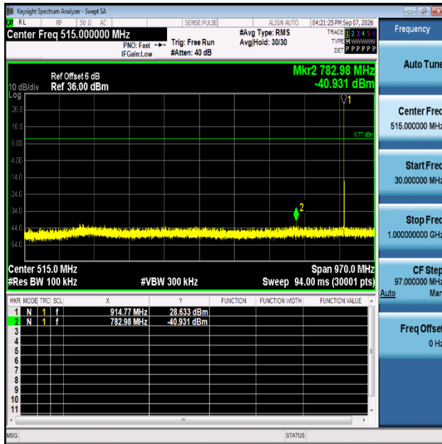
900M-Ant1-914.75-30~1000-PASS
