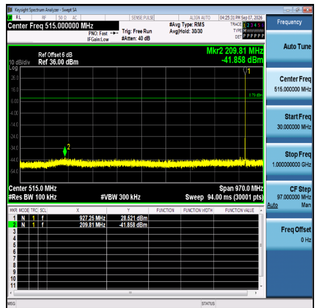
900M-Ant1-927.25-30~1000-PASS
