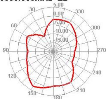
5300.000MHz E2
