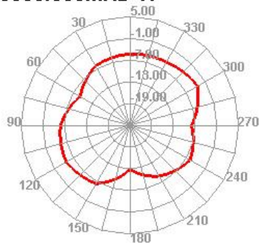
5300.000MHz H
