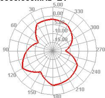
5300.000MHz E1
