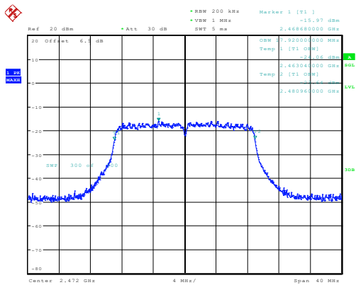
n20_2472MHz_Chain 0 17.920MHz
