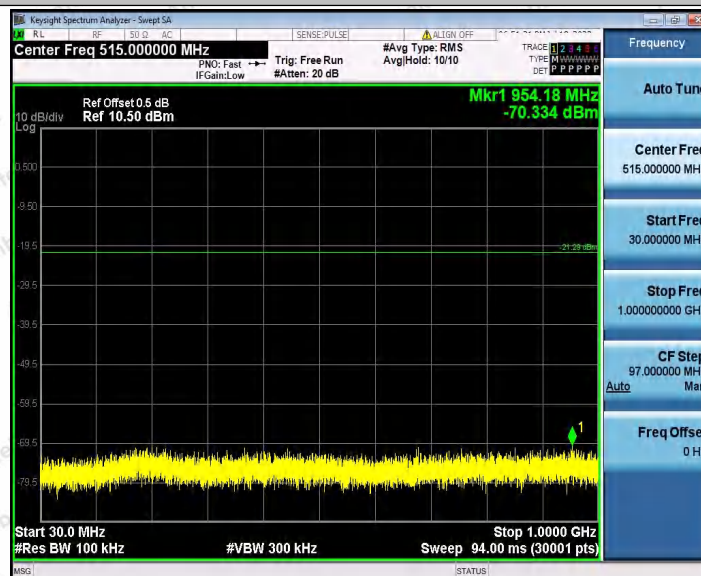
11N20_Ant1_2412_30~1000
