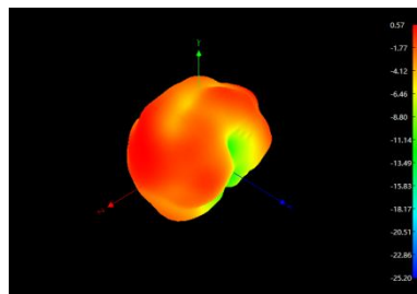
2450MHz
