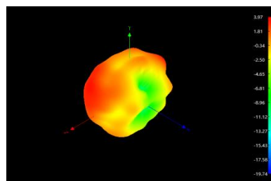
2500MHz
