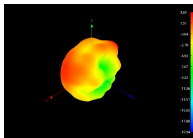
2500MHz
