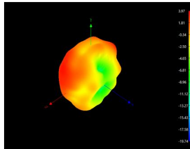
2500MHz
