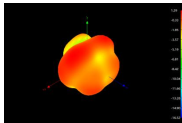
2400MHz
