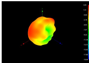
2450MHz
