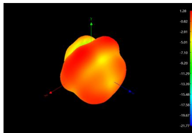
2450MHz
