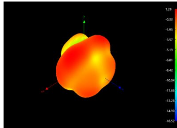
2450MHz
