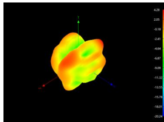
2500MHz
