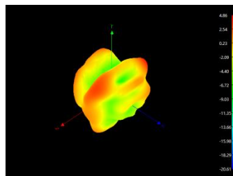
2450MHz
