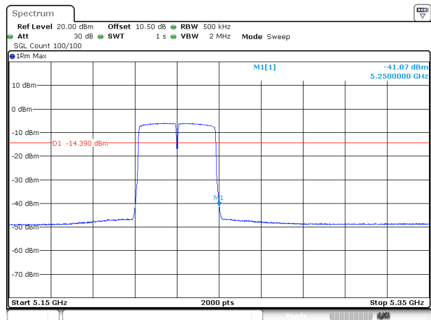
802.11ac40_5230MHz_Chain 0
