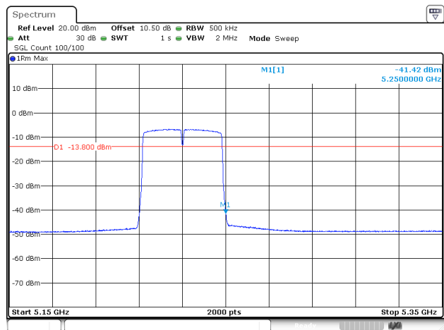
802.11ac40_5230MHz_Chain 1
