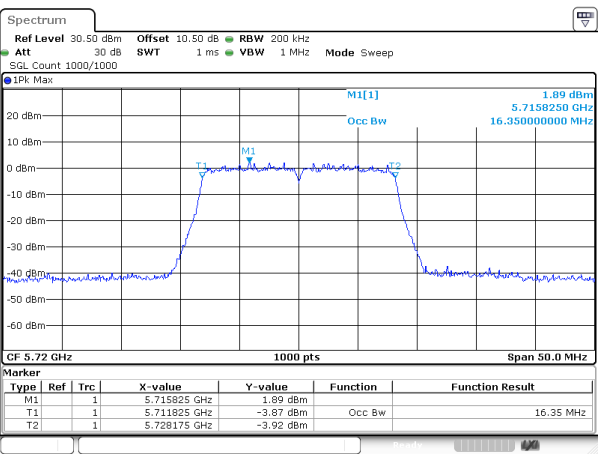
802.11a_5720MHz_Chain 0
