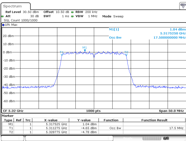
802.11ac20_5320MHz_Chain 0
