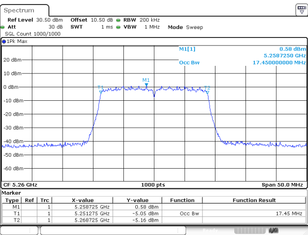
802.11ac20_5260MHz_Chain 1
