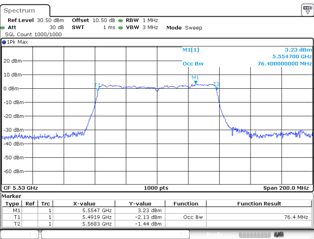
802.11ac80_5530MHz_Chain 1
