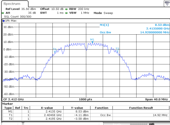
802.11b_2412MHz_Chain 0
