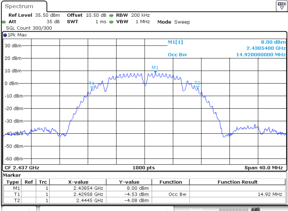
802.11b_2437MHz_Chain 0
