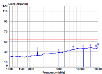
BLE_2M_TX_CH_39_Vertical-Avg
