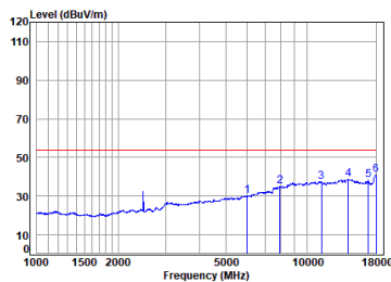
BLE_2M_TX_CH_39_Horizontal-Avg
