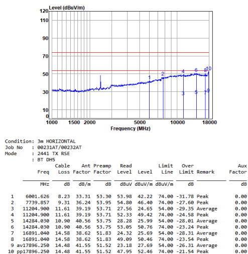
BT_DH5_TX_CH_39_Horizontal
