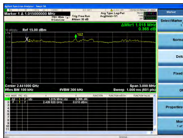
\pi/4 -DQPSK
