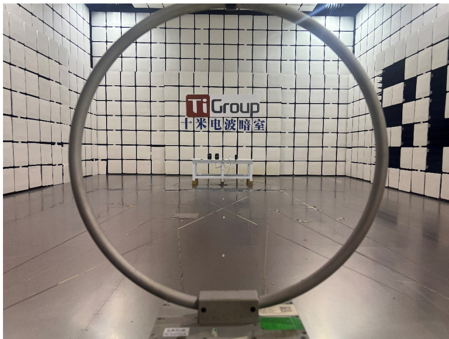
Below 30MHz-1.5m USB Cable
