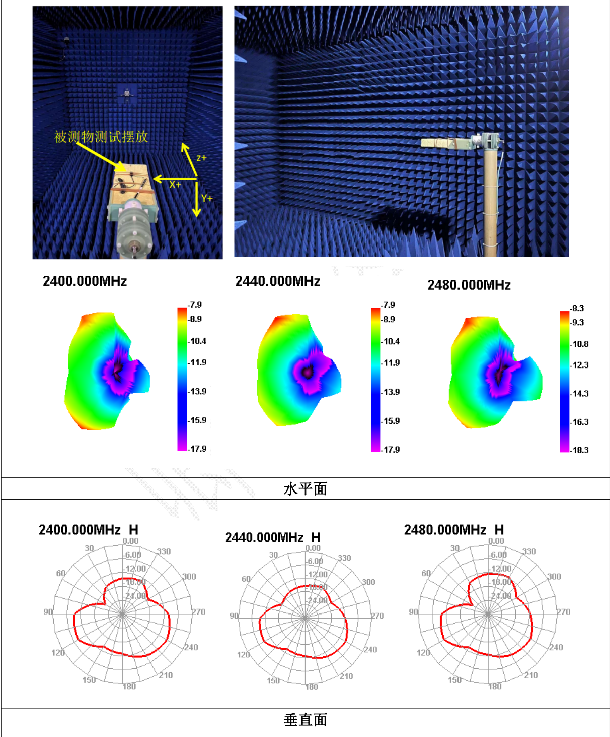
辐射方向图 (2.4G)
