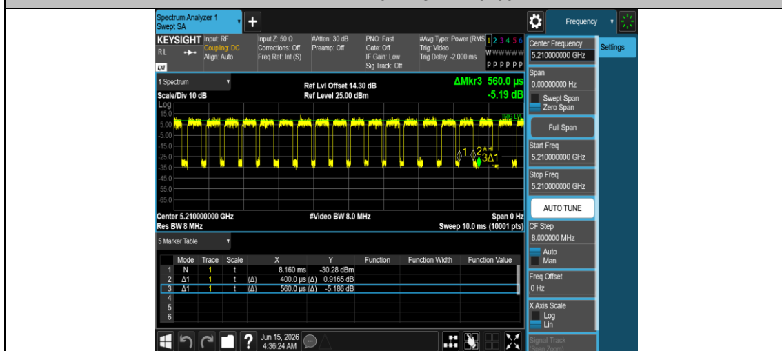
NTNV-11AX80MIMO-Ant1-5210
