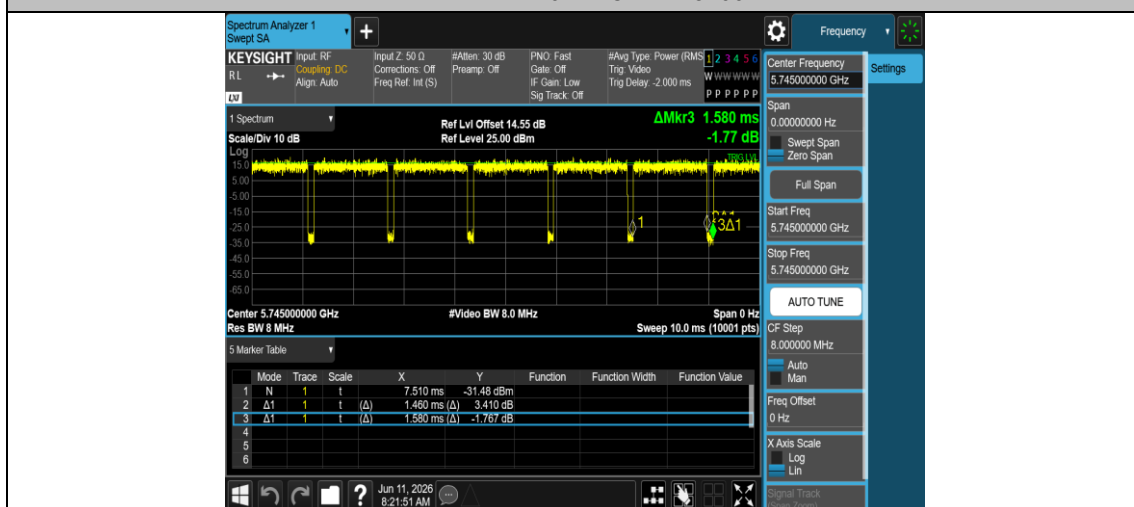
NTNV-11AX20MIMO-Ant1-5745
