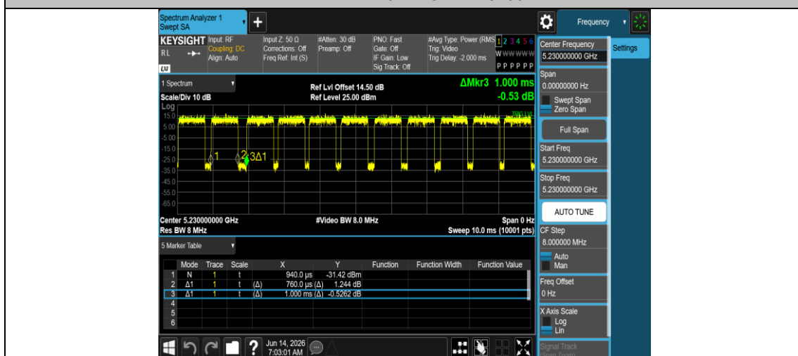
NTNV-11AX40MIMO-Ant2-5230
