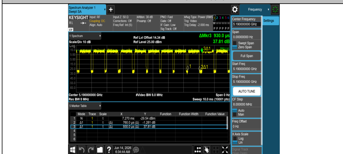
NTNV-11AX40MIMO-Ant1-5190
