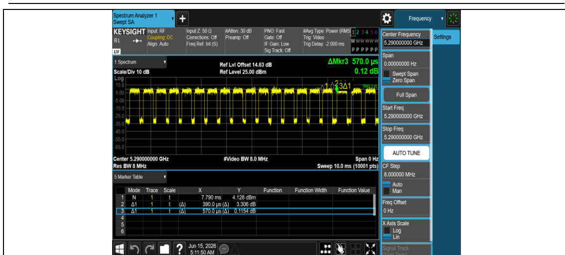
NTNV-11AX80MIMO-Ant1-5290
