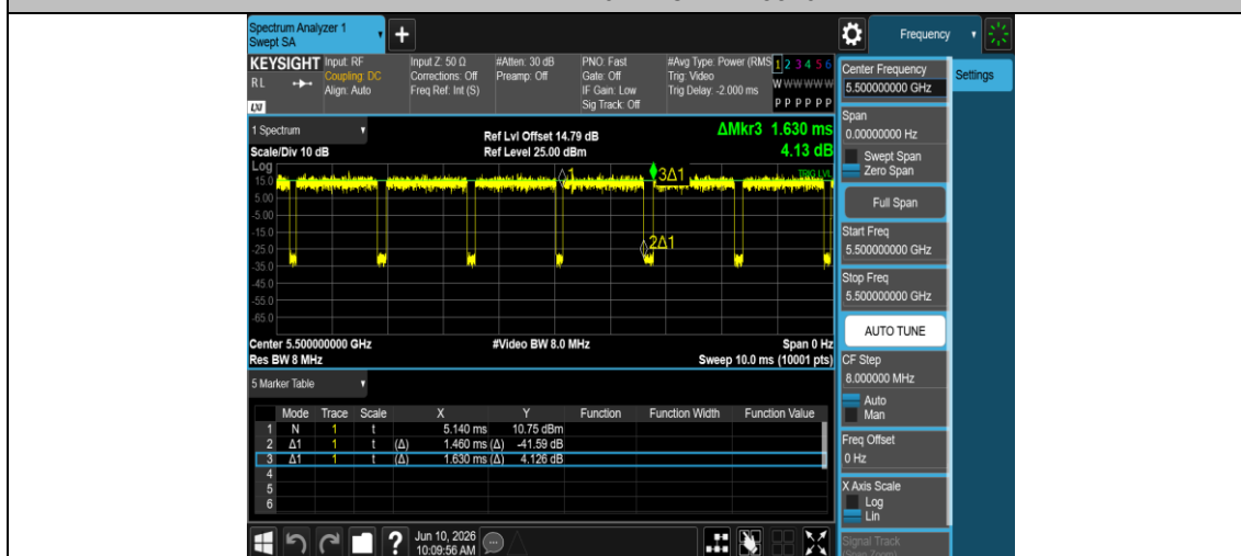
NTNV-11AX20MIMO-Ant1-5500
