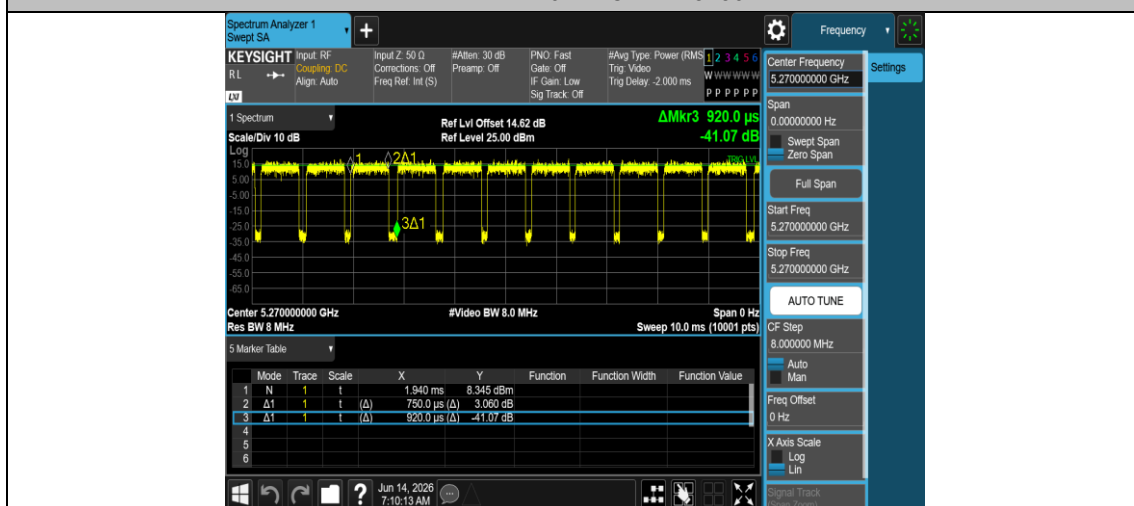
NTNV-11AX40MIMO-Ant1-5270
