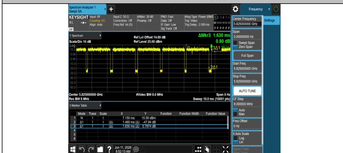
NTNV-11AX20MIMO-Ant1-5825
