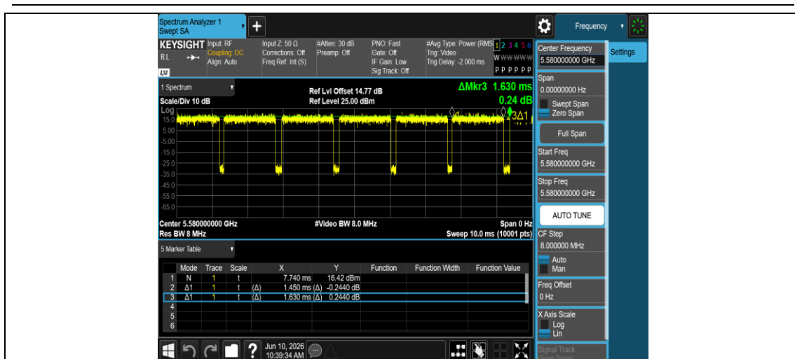
NTNV-11AX20MIMO-Ant1-5580
