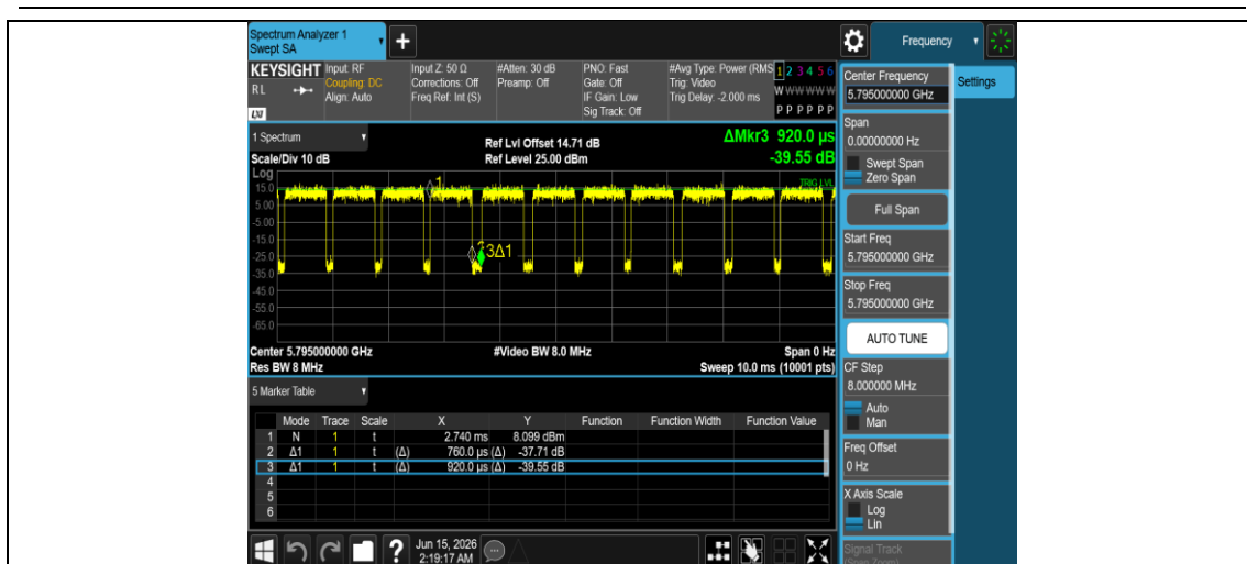
NTNV-11AX40MIMO-Ant2-5795
