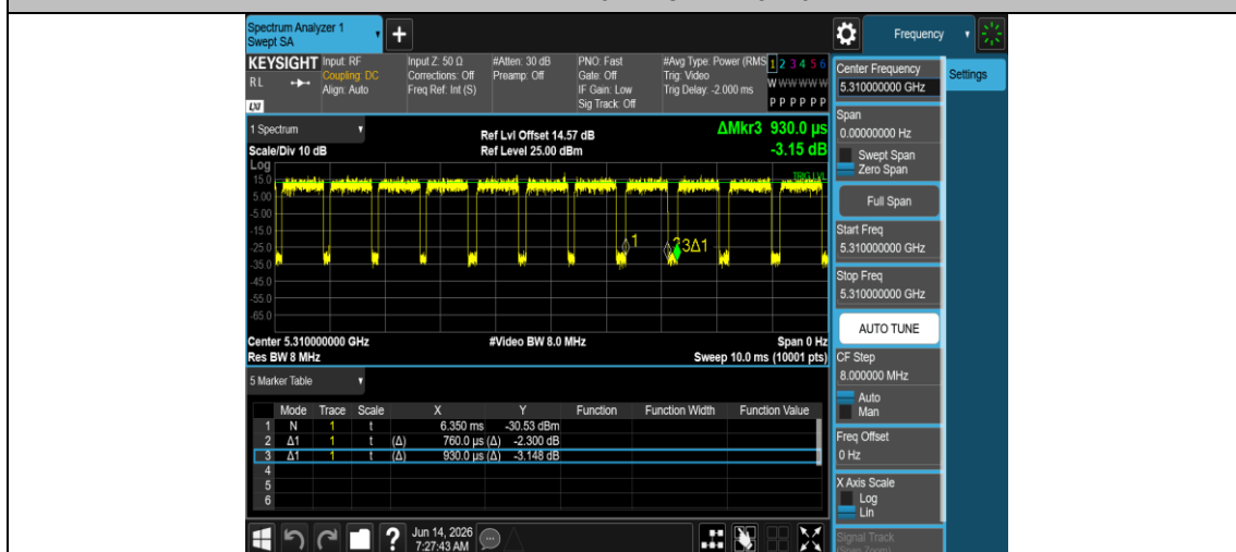
NTNV-11AX40MIMO-Ant1-5310
