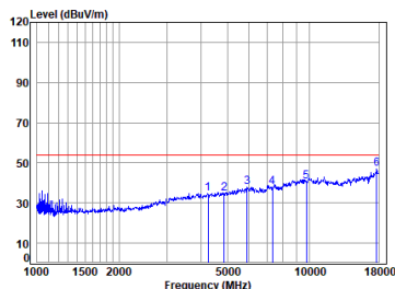
11n_HT(20M)_TX_CH_06_Horizontal-Avg
