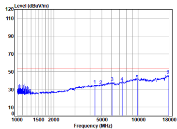
11n_HT(20M)_TX_CH_11_Vertical-Avg
