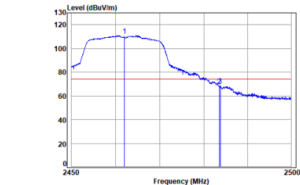
11n_HT(20M)_TX_CH_11_Horizontal-Peak
