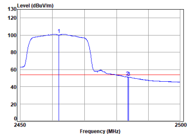
11n_HT(20M)_TX_CH_11_Horizontal-Avg
