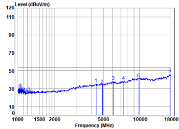
11ax_20M_TX_CH_11_Horizontal-Avg
