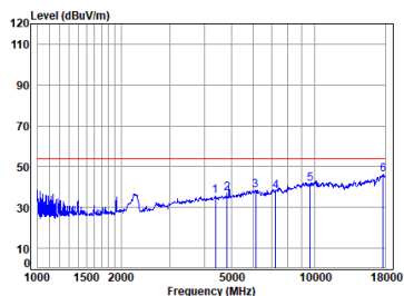
11b_TX_CH_01_Horizontal-Avg
