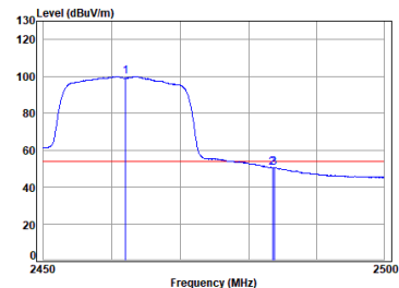
11n_HT(20M)_TX_CH_11_Vertical-Avg
