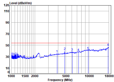
11b_TX_CH_06_Vertical-Avg
