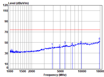
11n_HT(20M)_TX_CH_11_Horizontal-Peak
