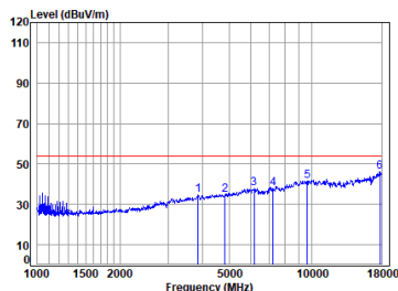
11ax_20M_TX_CH_01_Horizontal-Avg
