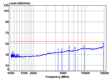
11ax_20M_TX_CH_06_Horizontal-Avg
