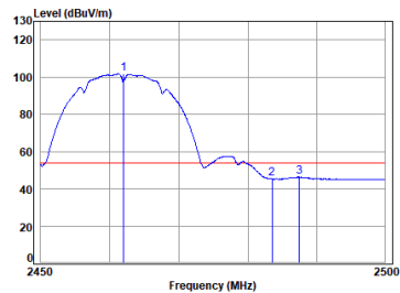
11b_TX_CH_11_Vertical-Avg
