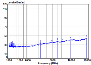
11ax_20M_TX_CH_11_Vertical-Avg
