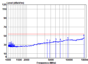
11ax_20M_TX_CH_01_Vertical-Avg
