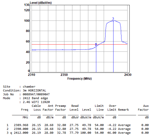
11n_HT(20M)_TX_CH_01_Horizontal-Avg
