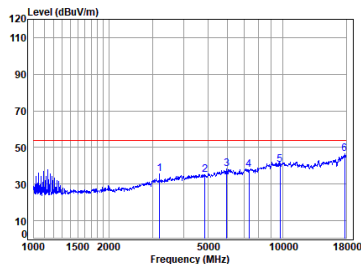
11n_HT(20M)_TX_CH_06_Vertical-Avg
