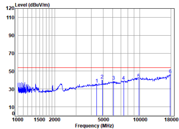
11b_TX_CH_11_Vertical-Avg
