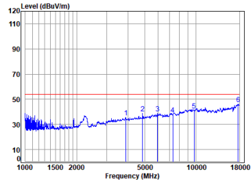
11b_TX_CH_06_Horizontal-Avg
