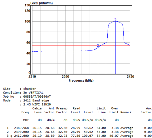
11n_HT(20M)_TX_CH_01_Vertical-Avg
