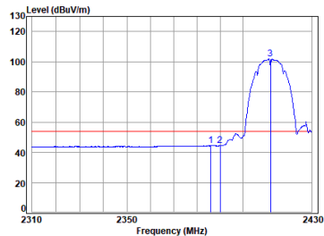
11b_TX_CH_01_Vertical-Avg
