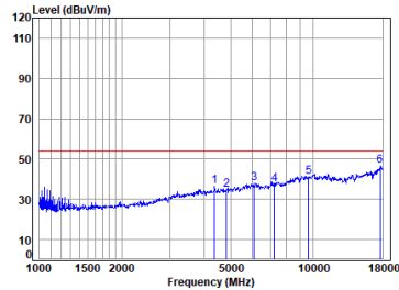
11n_HT(20M)_TX_CH_01_Horizontal-Avg
