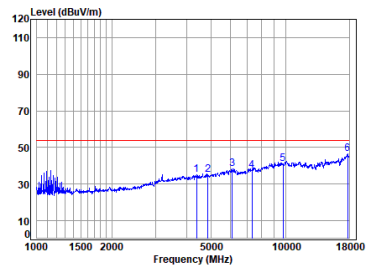
11ax_20M_TX_CH_06_Vertical-Avg
