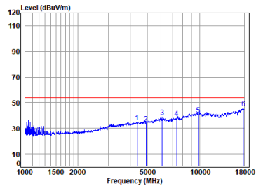
11n_HT(20M)_TX_CH_11_Horizontal-Avg
