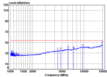
11n_HT(20M)_TX_CH_01_Vertical-Avg
